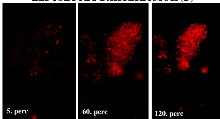
5. ábra. Fotokatalizátor szemcséken adszorbeálódott Pseudomonas aeruginosa baktériumok. A jelző festék egyik komponense az élő baktériumokhoz (A), míg a másik komponens az elpusztult baktériumokhoz kapcsolódik (B).
