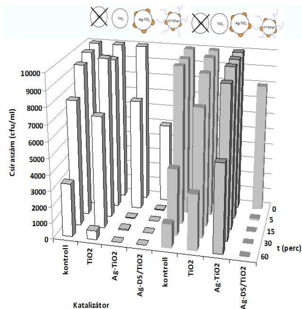
3. ábra. A P25 \text{TiO}_2 , Ag- \text{TiO}_2 és Ag-DS/ \text{TiO}_2 felületi katalizátort tartalmazó festék alapú filmekken meghatározott csíraszámok látható fényel történő bevilágítás mellett Staphylococcus aureus ATCC ( S.aureus ) Gram (+) baktériumok (világos oszlopok), valamint Pseudomonas aeruginosa ATCC 27853 Gram (-) baktériumok (sötét oszlopok) esetében
